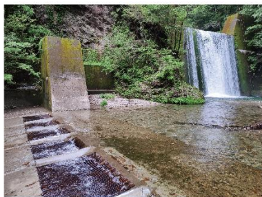
小又川小水力発電所 取水口
